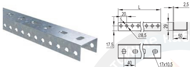
а) Профиль BPM-29
