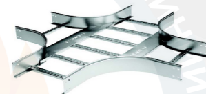
Х-образный ответвитель R300
