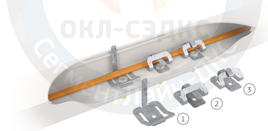
Последовательность закрепления кабеля хомутом FR ПР
