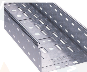
Перфорированные лотки с высотой борта 100мм
