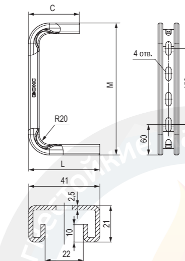
Консоль потолочная BBA-30 (DS)
