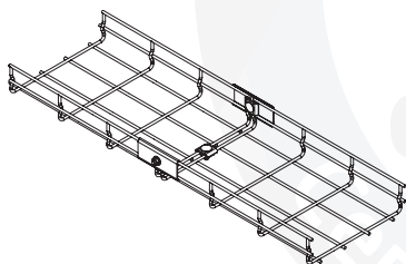
Соединение лотков с помощью пластин с отверстиями
