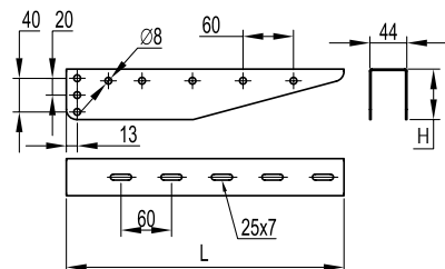
Консоль ВВМ-50 (ВМ 200-60)
